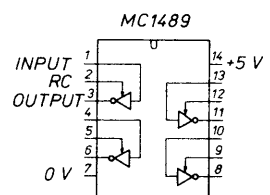
Obr. 4. Zapojení vývodů MC1488 a MC1489
